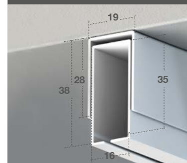
guida telescopica
